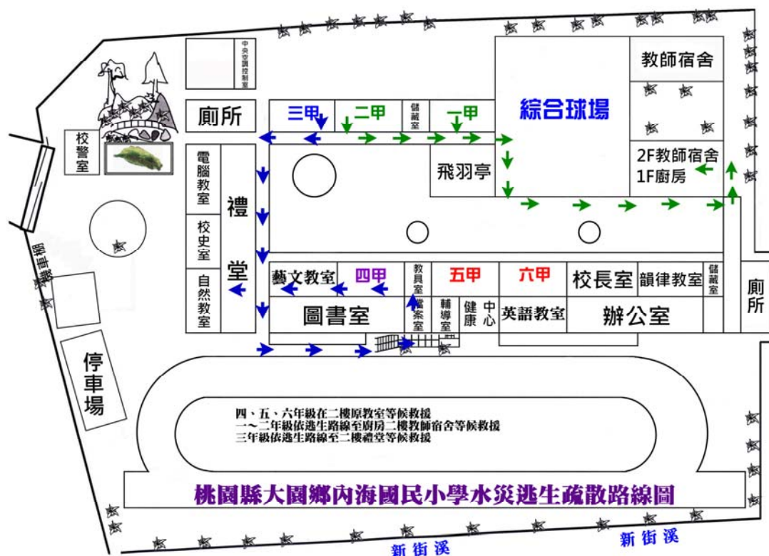
圖 4-2-4 避難、疏散路線圖
